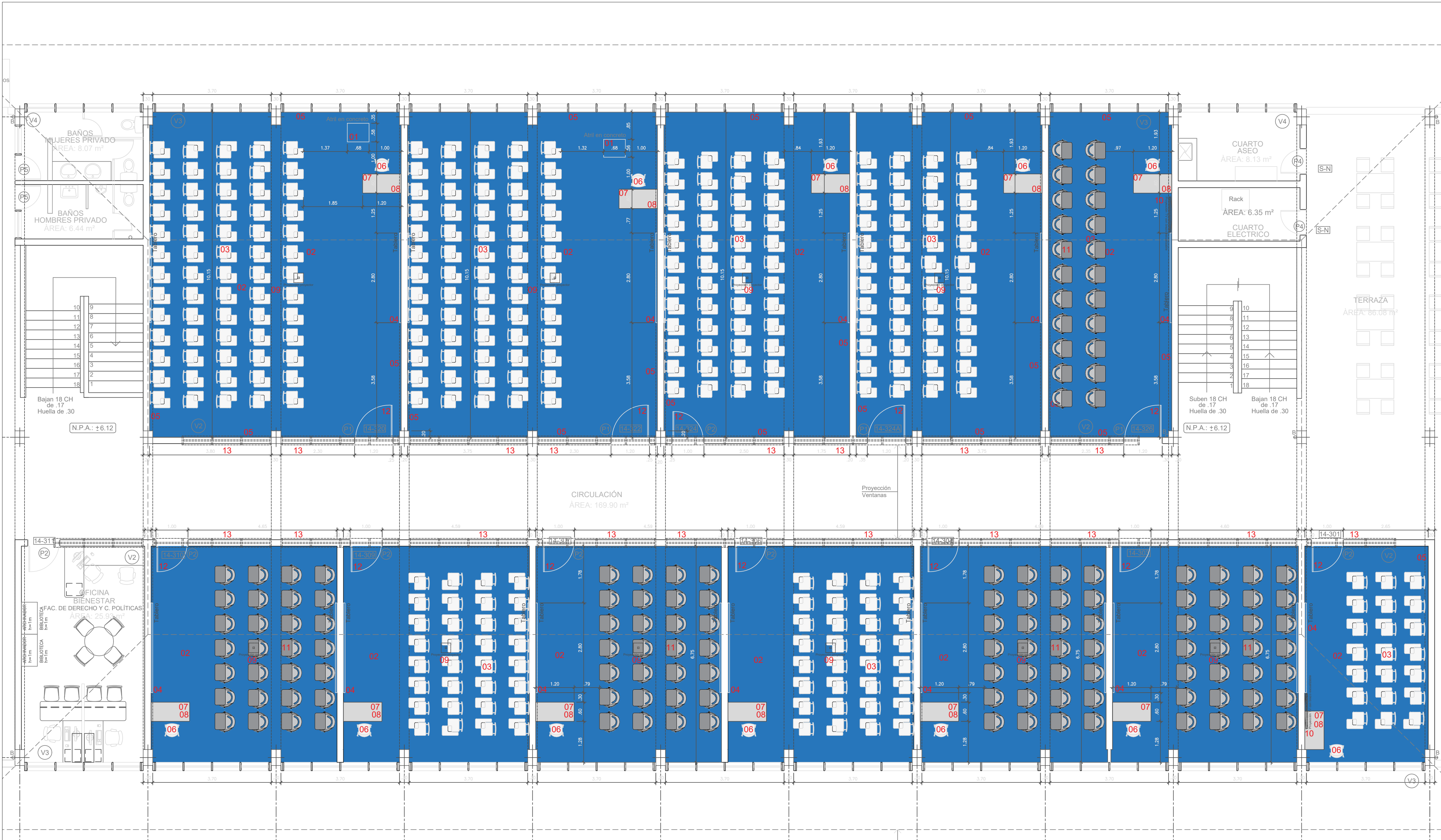
PLANTA TERCER PISO, BLOQUE 14 - AULAS PARA INTERVENCIÓN ESC. 1:75
