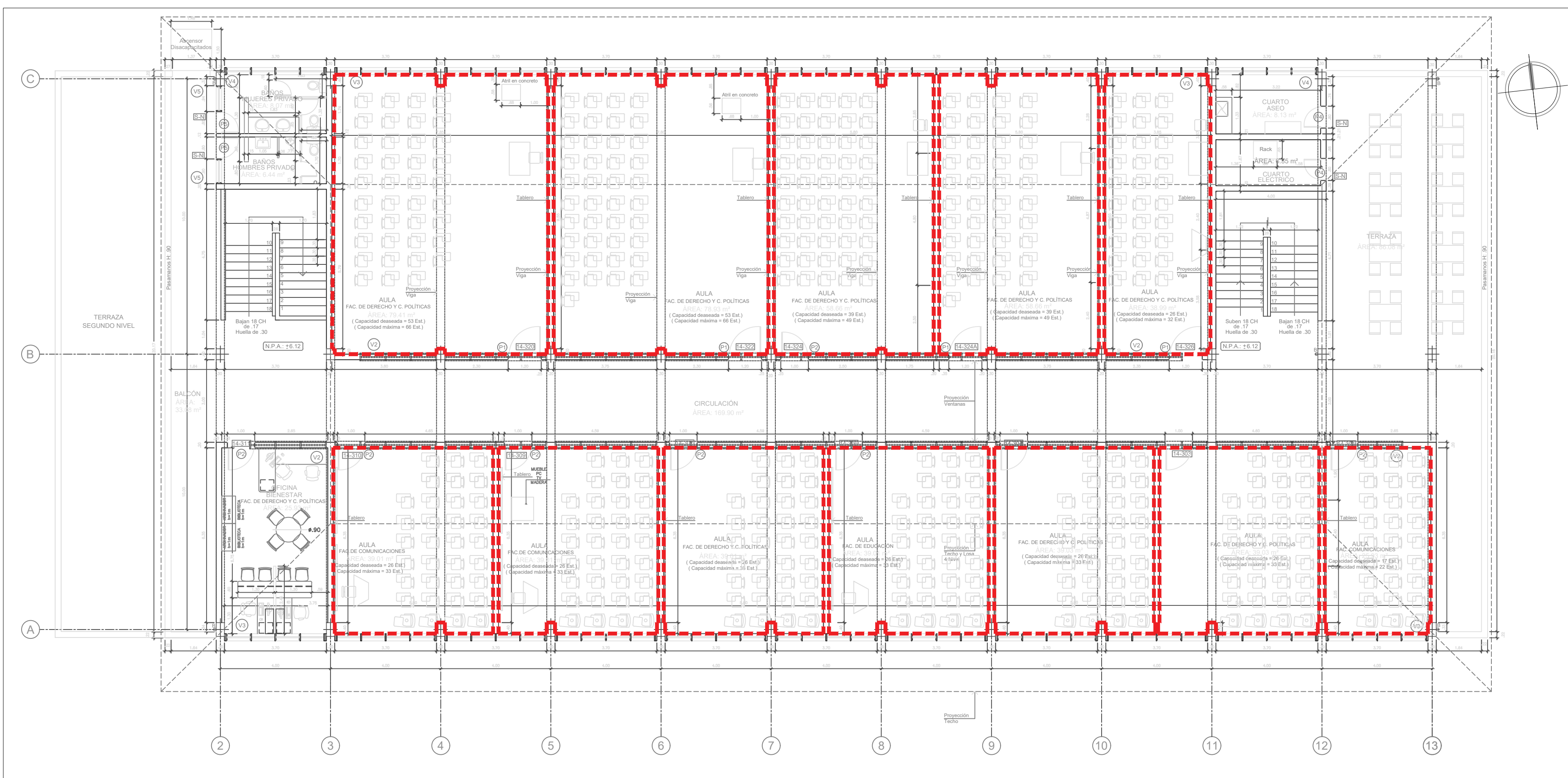
PLANTA TERCER PISO, BLOQUE 14 - ESTADO ACTUAL. ESC. 1:100
